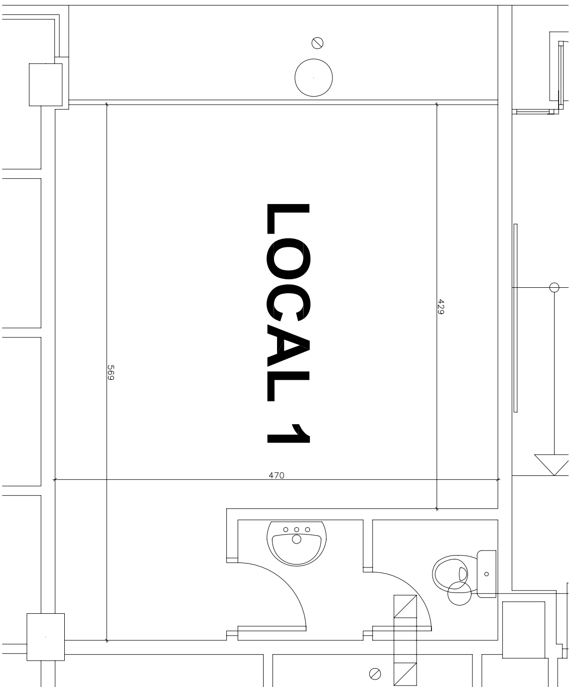
PLANTA LOCAL 1 ESCALA GRAFICA 1/40
